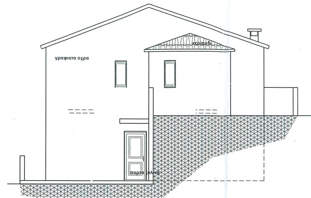
ΠΡΟΣΟΨΗ
