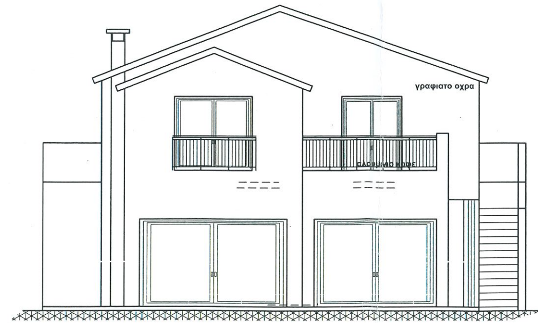
ΠΙΣΩ ΟΨΗ
